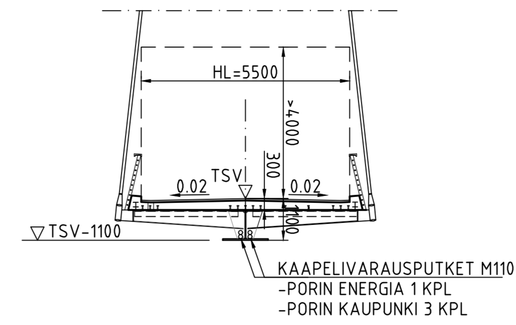
B - B 1:100
