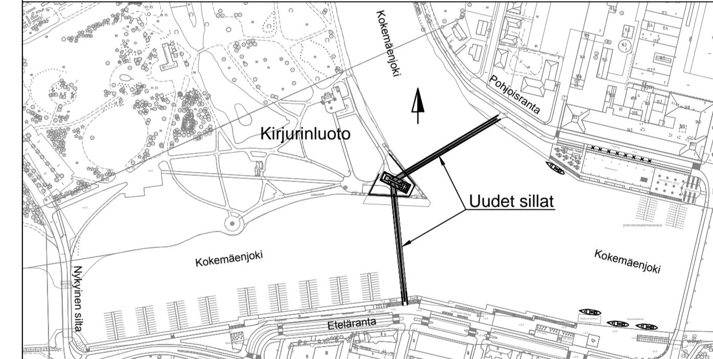
SILTAPAIKAN KARTTA 1:5000
