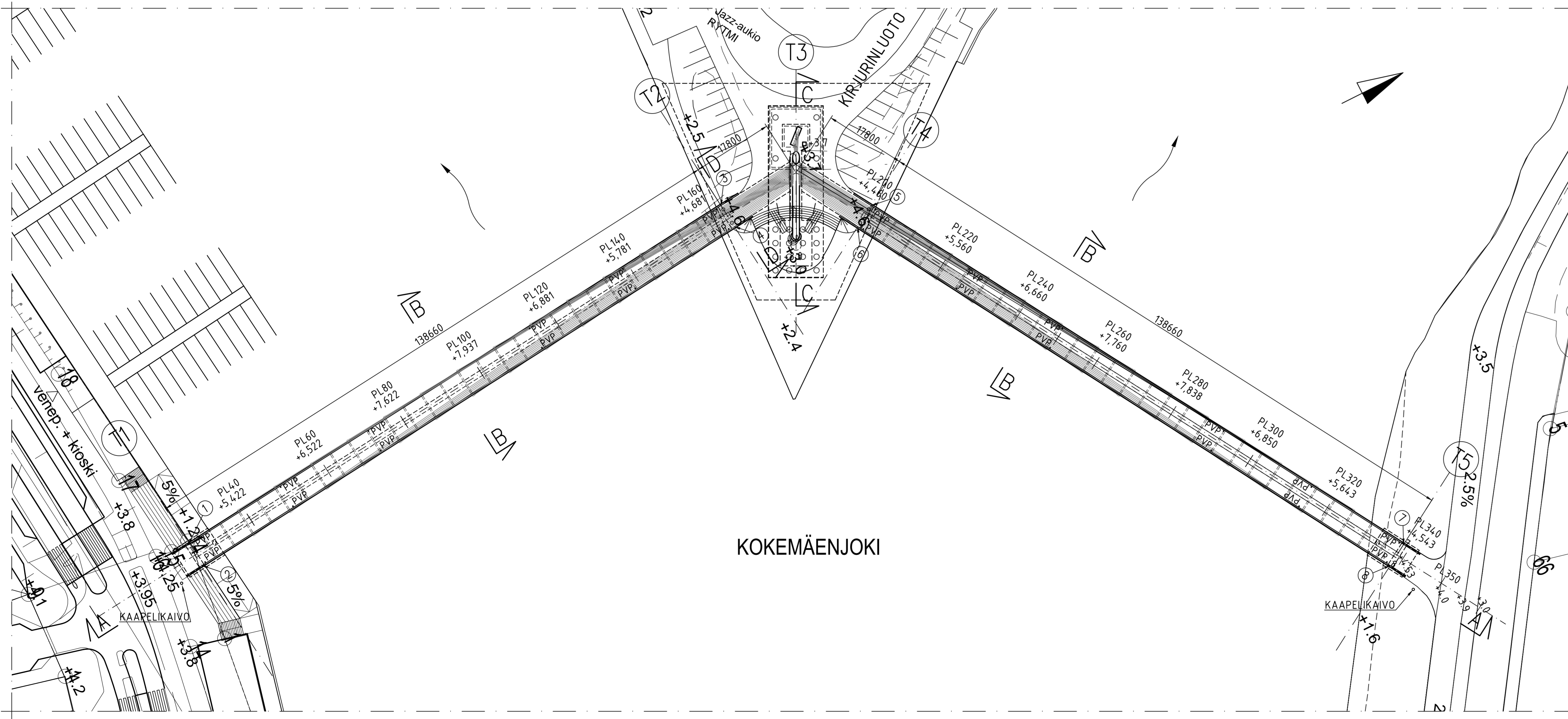
TASOPIIRUSTUS 1:500
