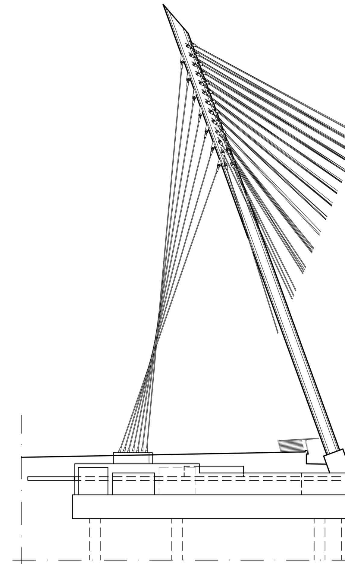
C - C 1:250
