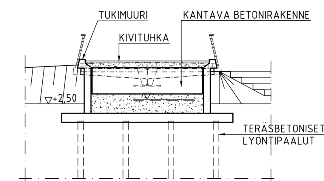
D - D 1:100
