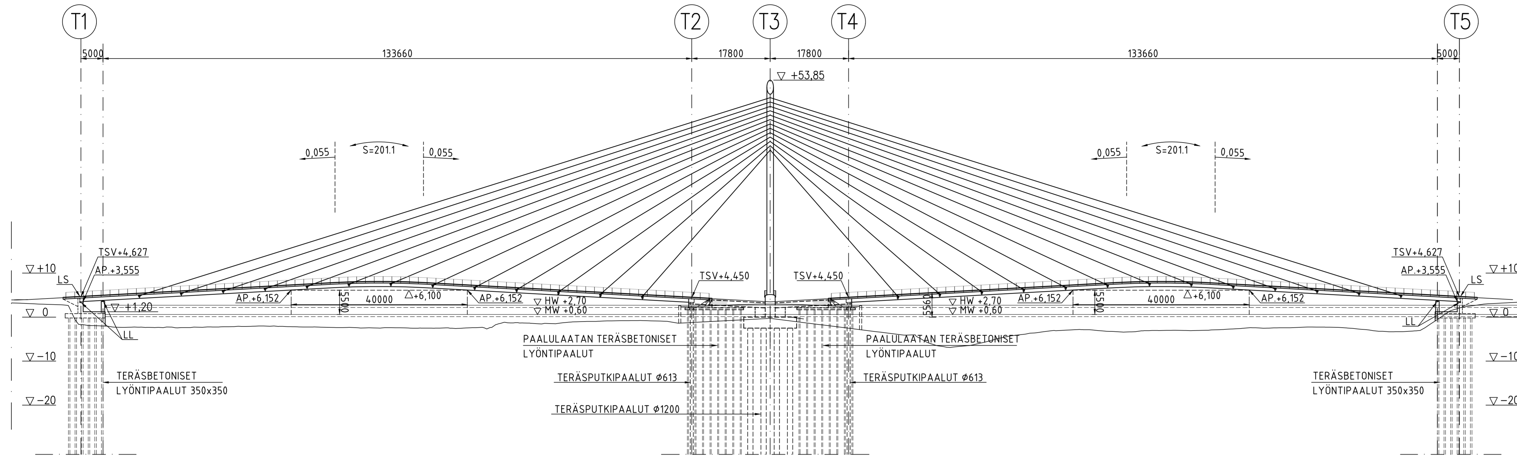
A - A 1:500
