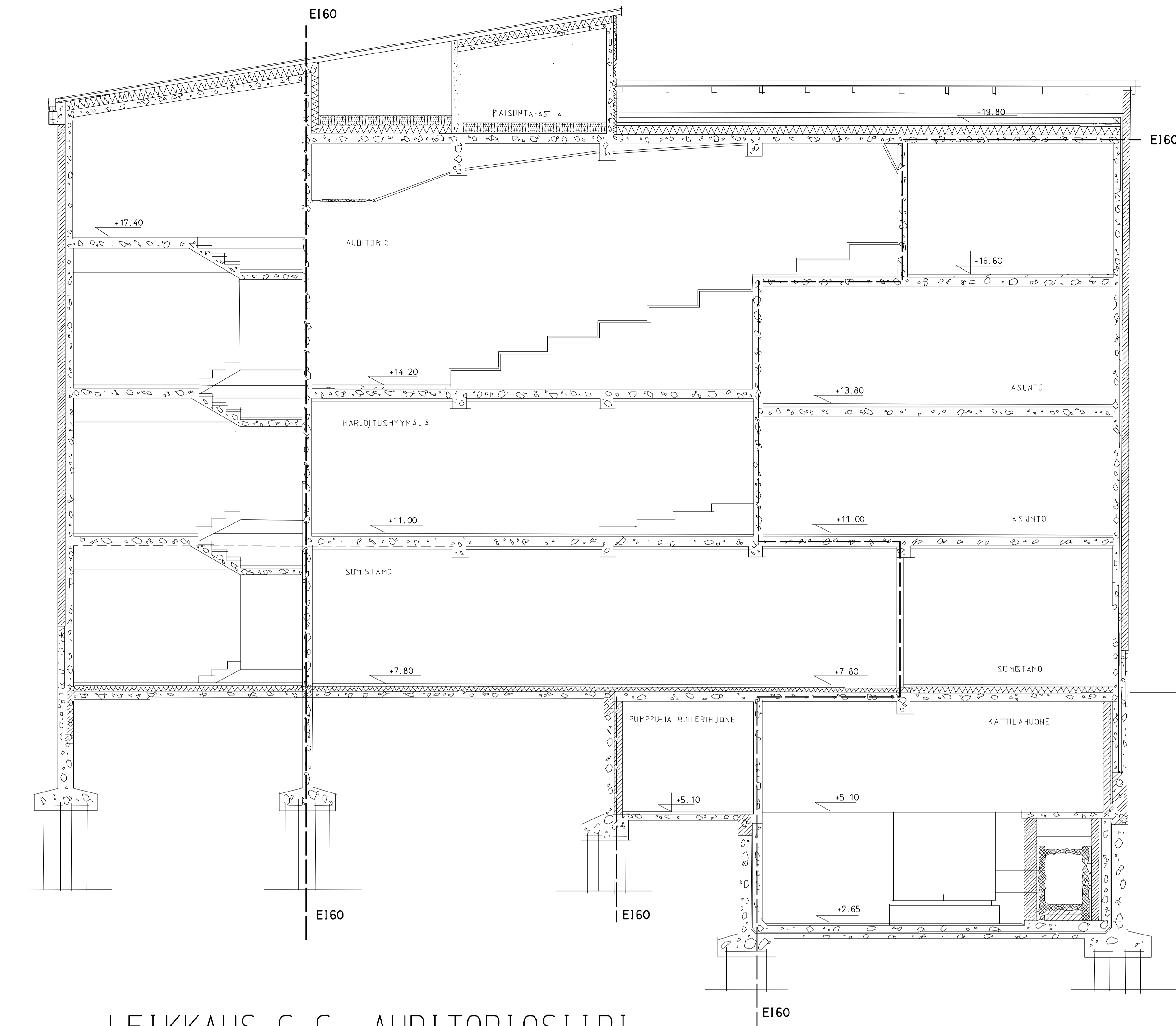
LEIKKAUS C-C AUDITORIOSIIPPI
