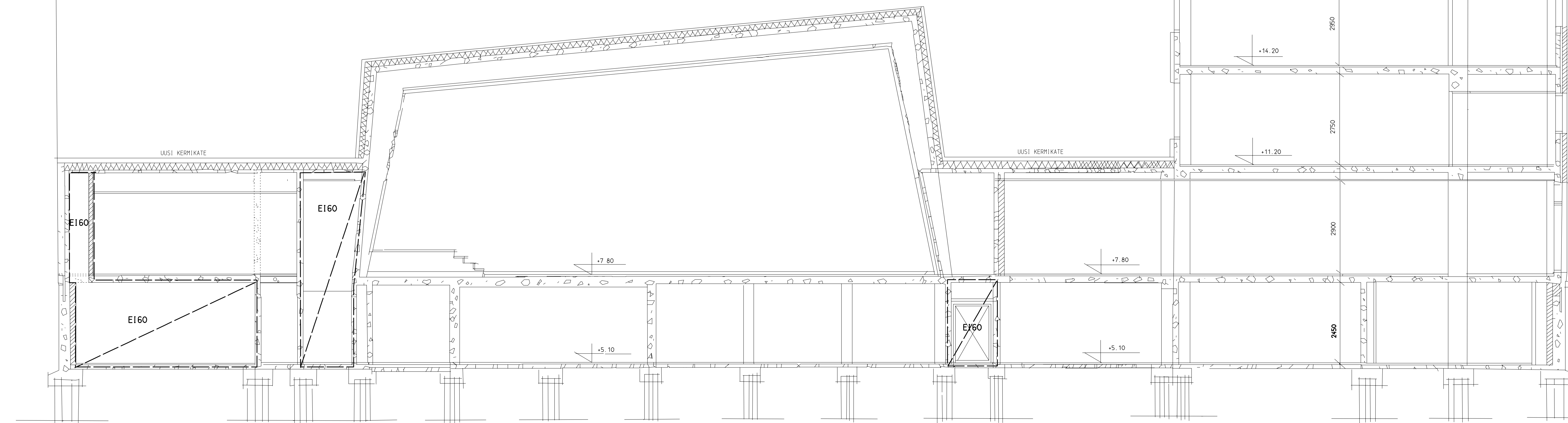
LEIKKAUS A-A JUHLASALI JA KEITTIÖ
