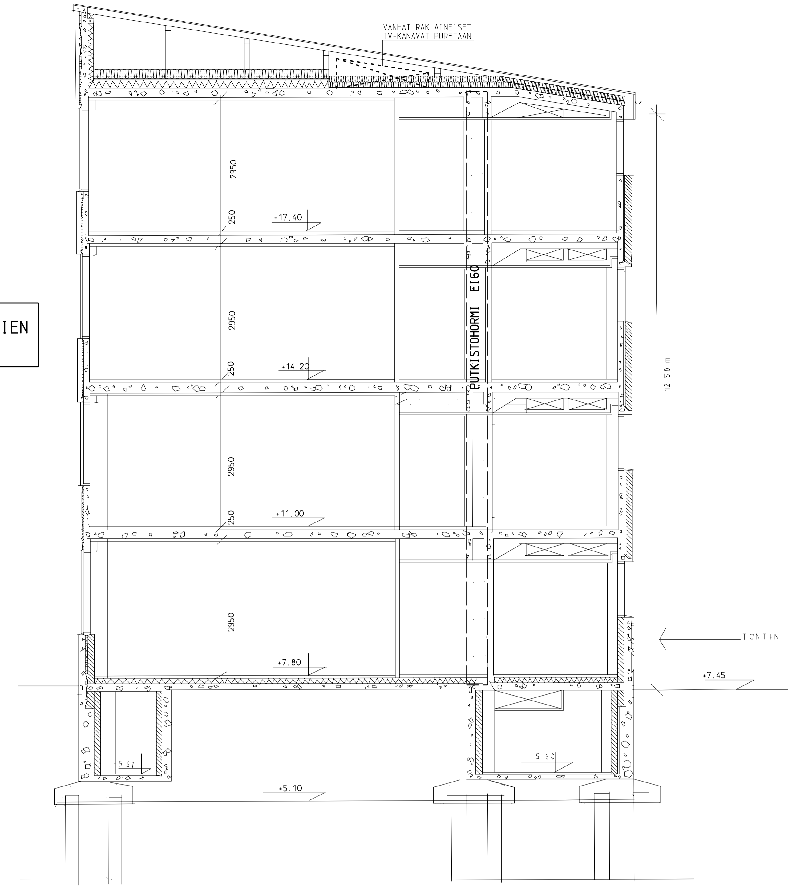
LEIKKAUS B-B KESKIOSA
